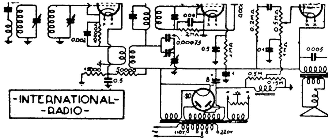
IRRADIO. — Mod. Folletto. — Valvole e valori indicati. — MF: 175 kHz. — Produzione 1933-1934.
